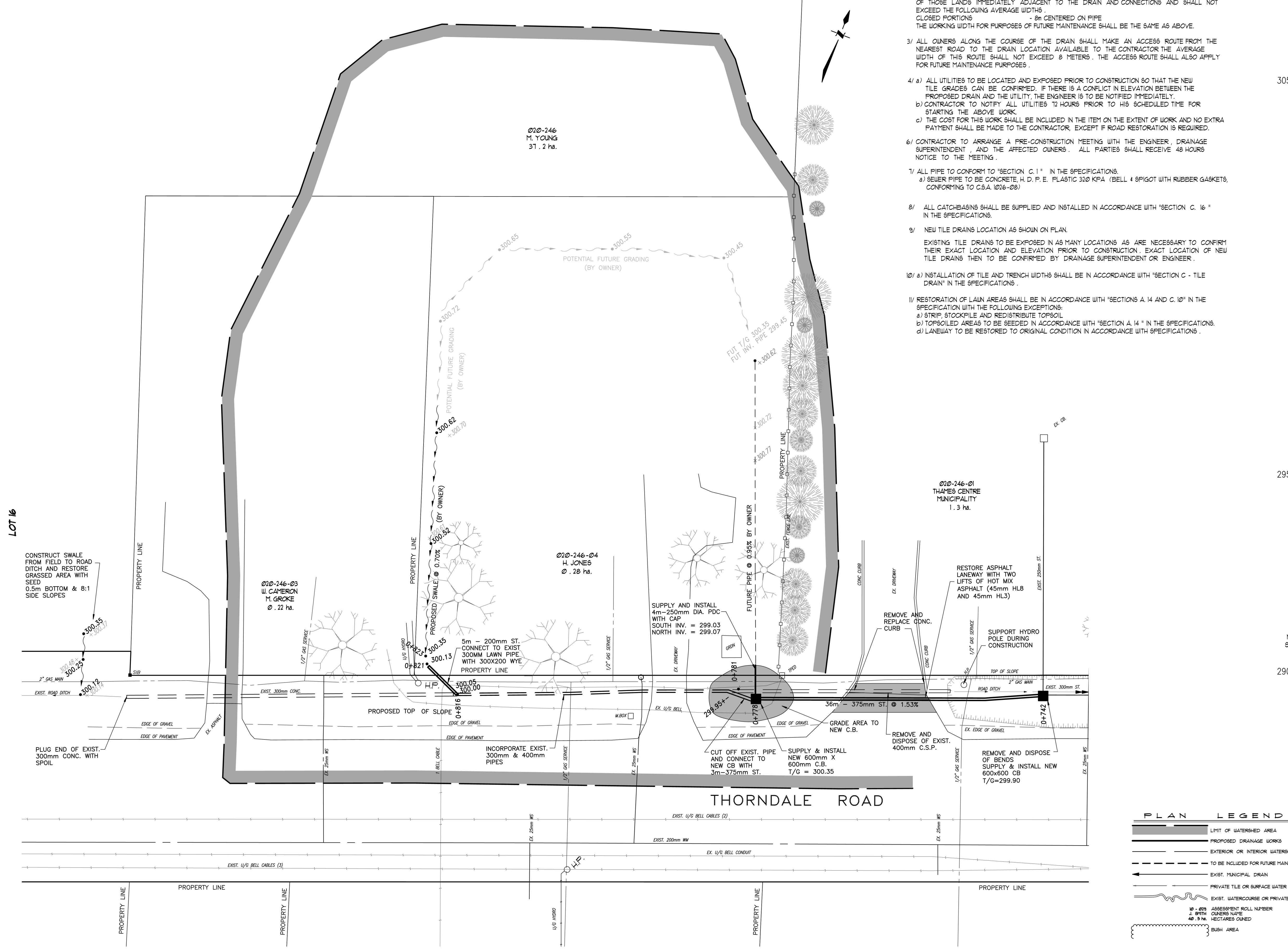
PLAN SCALE 1 : 250
